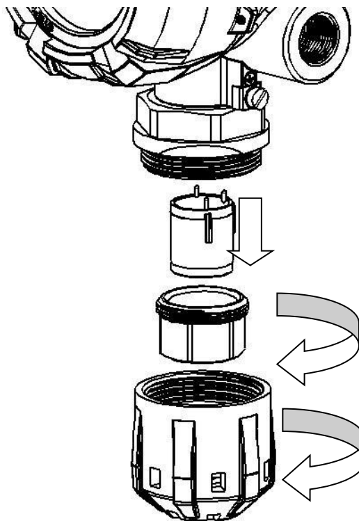
Рисунок 56 – Схема разборки газоанализатора
