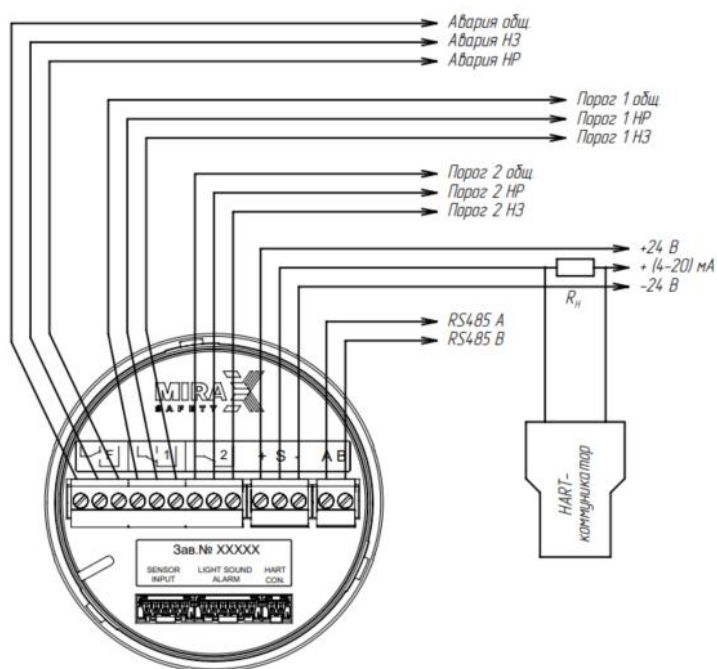
Рисунок 30 – Схема подключения газоанализатора AXIOM
