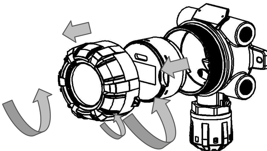
Рисунок 29 – Схема разбора AXIOM
