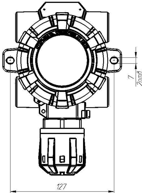
Рисунок 33 – Монтажные размеры
