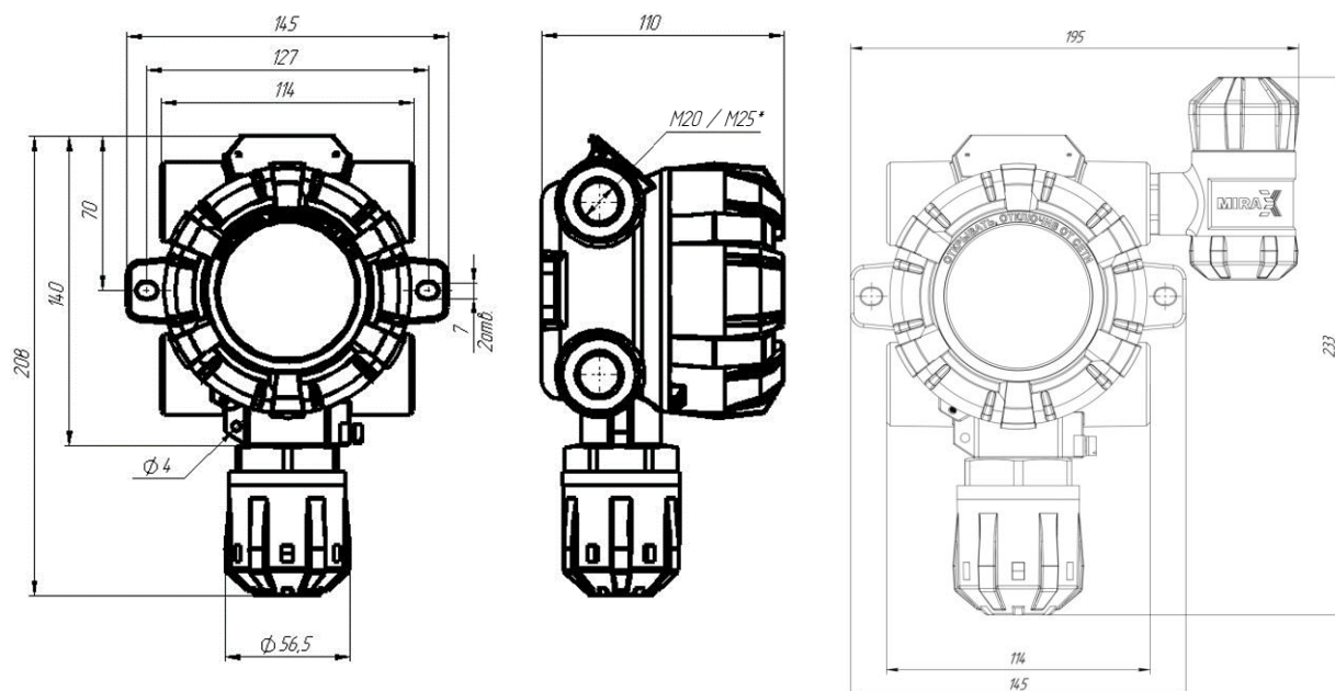
Рисунок 4 – Габаритные размеры AXIOM
