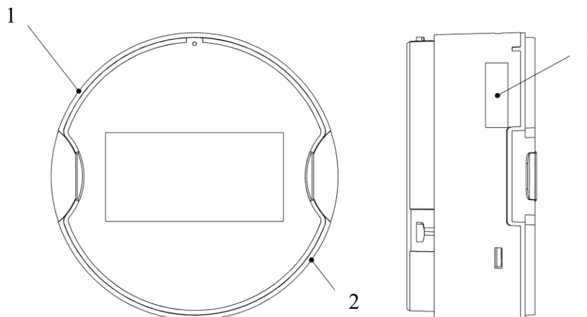
Рисунок 7 - Расположение гарантийных наклеек на электронном модуле газоанализатора 1,2 - гарантийные наклейки
